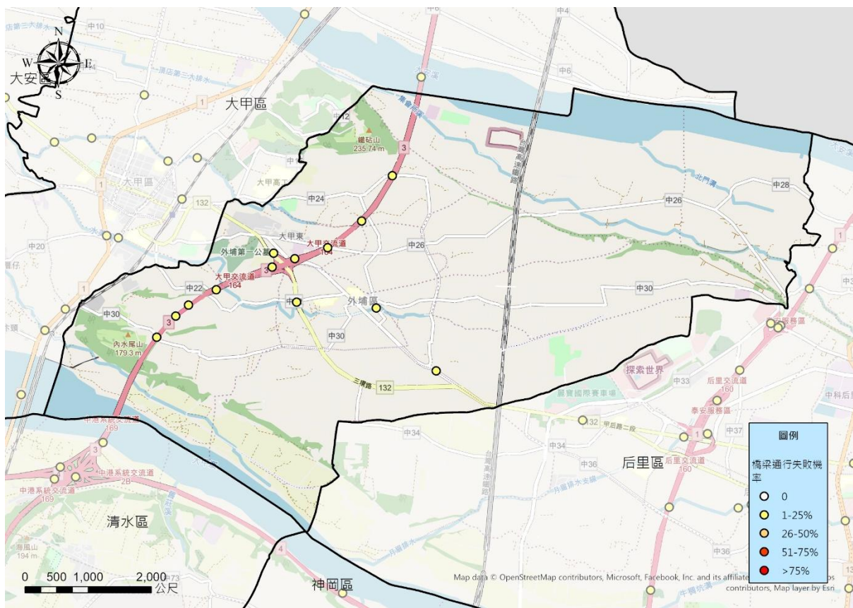
圖 1-6 本區受損橋梁分布圖
