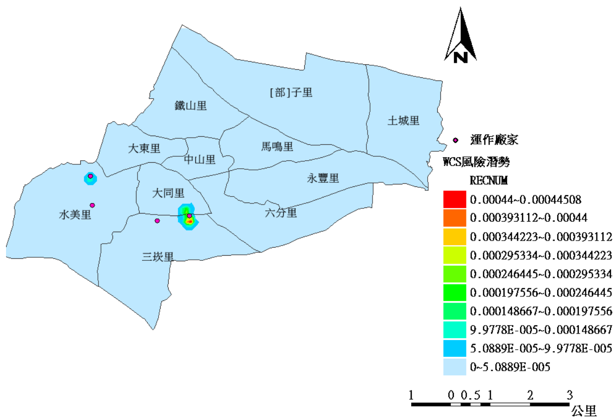
圖 5-3 臺中市外埔區最嚴重洩漏模擬情境(WCS)毒性及關注化學物質災害潛勢圖
