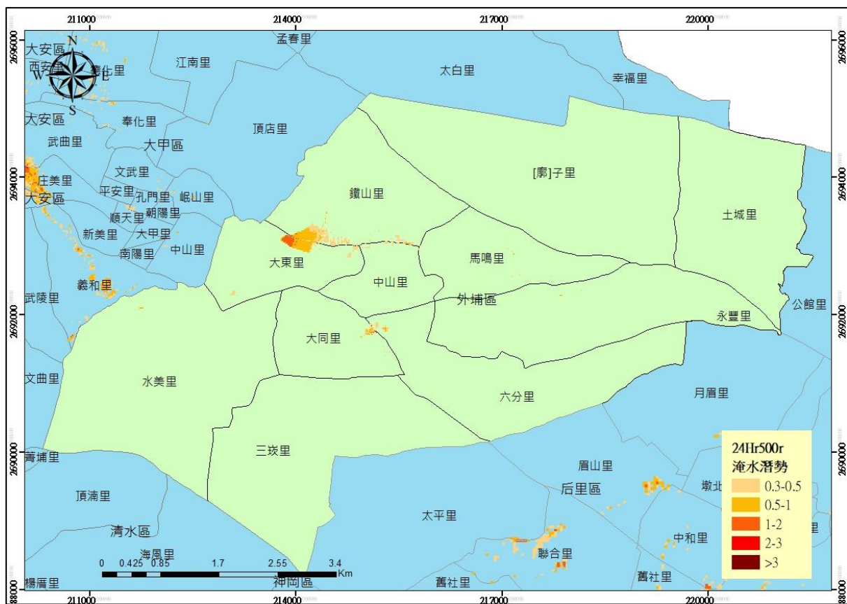
圖 2-7 外埔區 24 小時累積 500 毫米淹水潛勢圖
