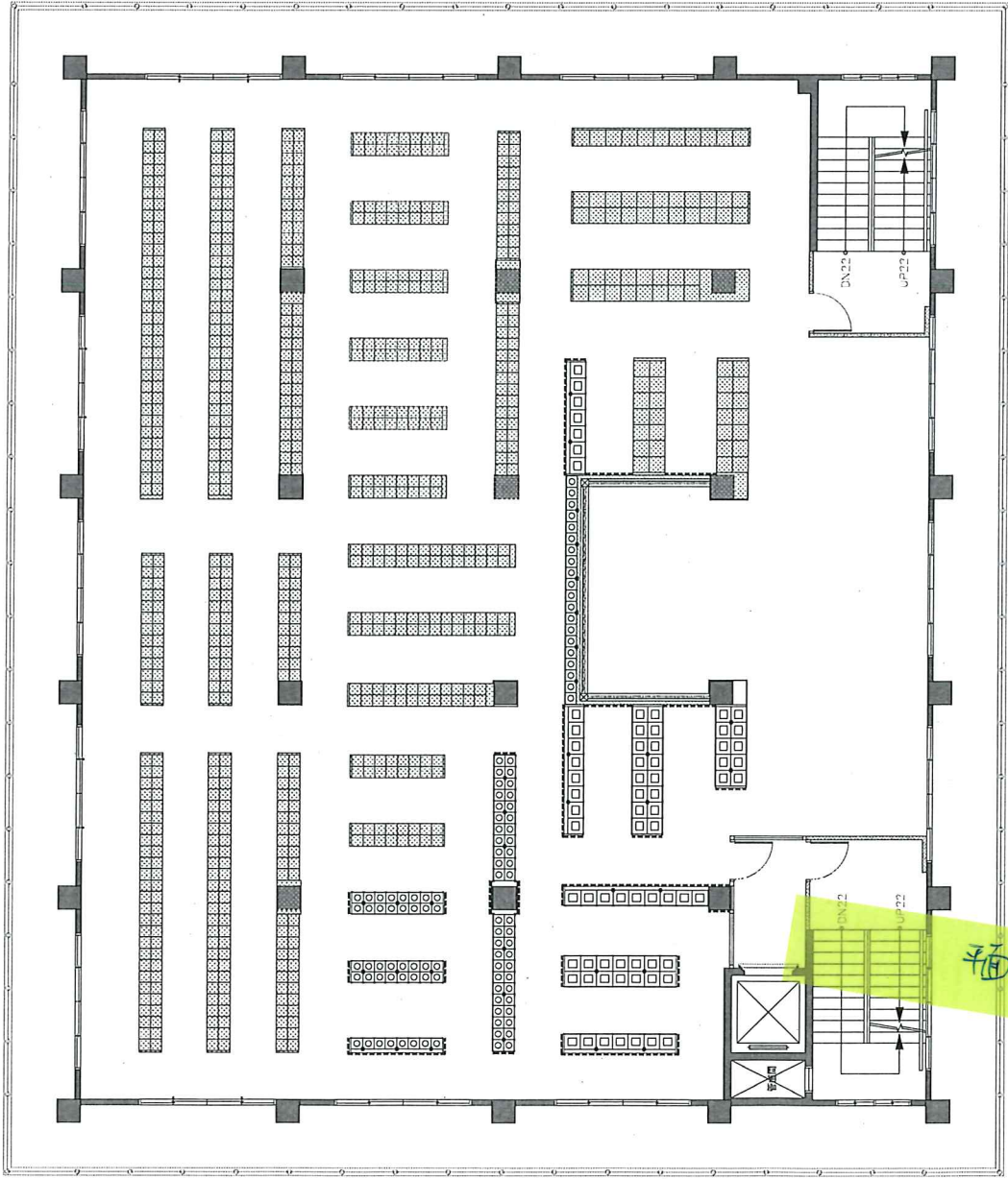
1 五樓裝修平面圖 SCALE 1:1/65 A3:1/130
